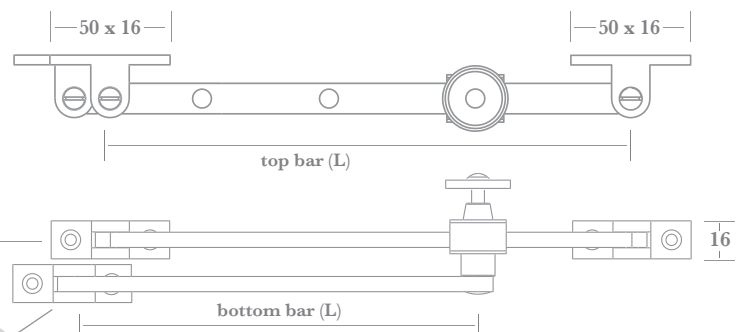
8023 & 8027 INWARD opening windows
