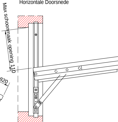
Horizontale Doorsnede
