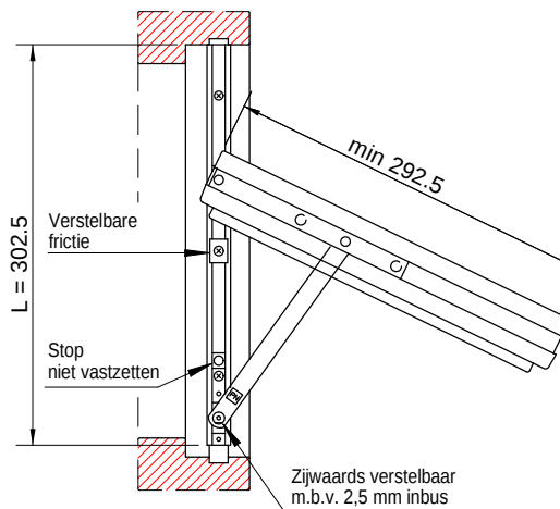
Horizontale Doorsnede
