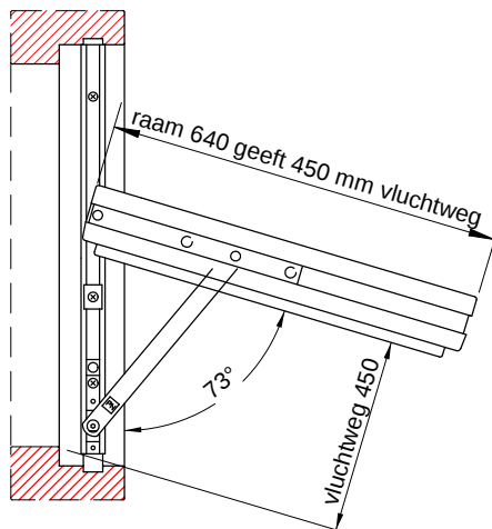
Horizontale Doorsnede
